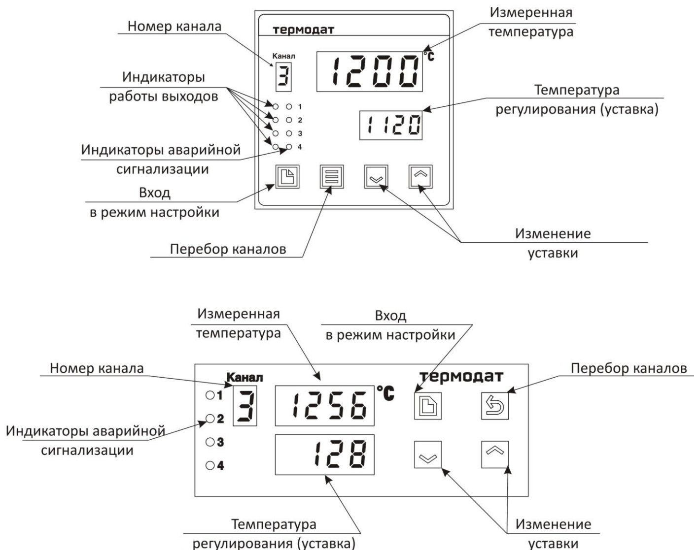
Рисунок 2 – Описание индикаторов и кнопок управления приборов
