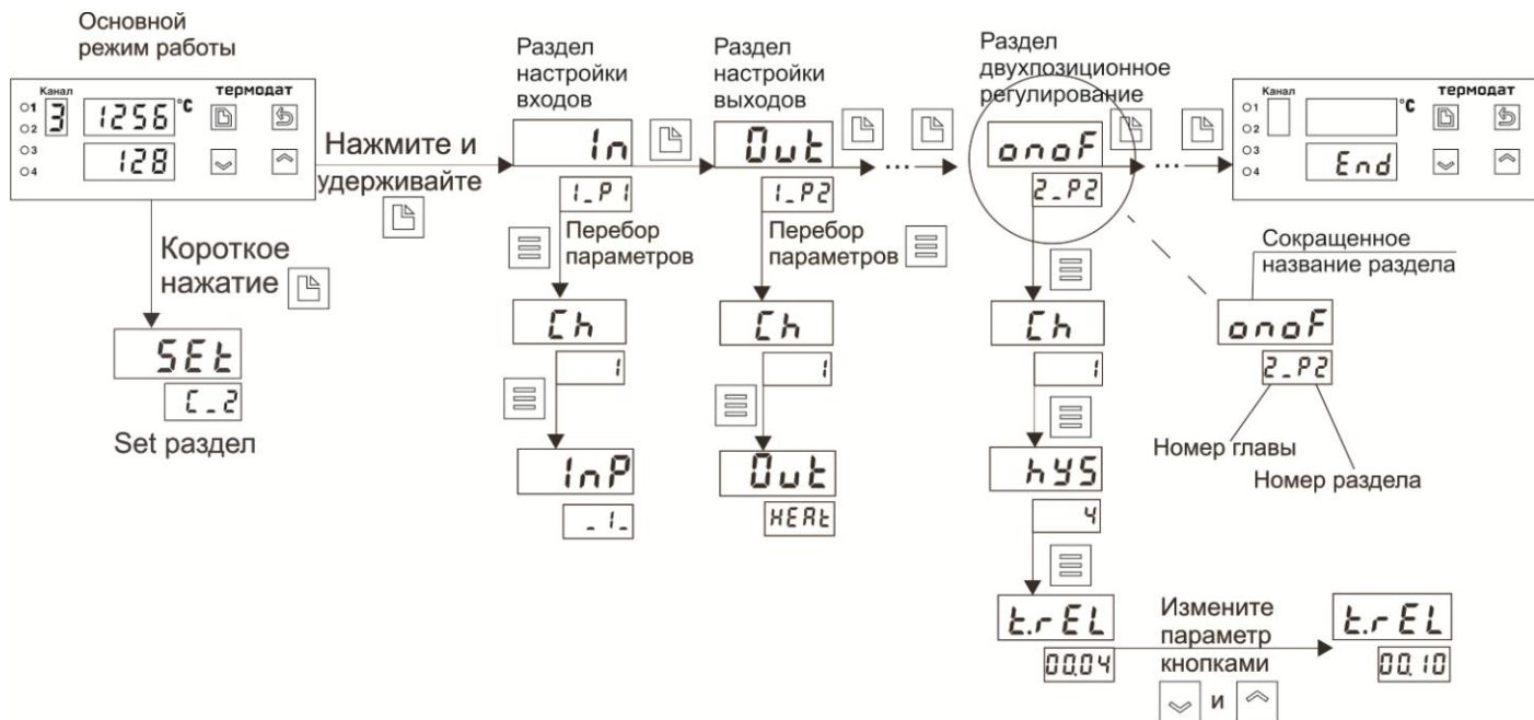
Рисунок 3—Схема меню настройки прибора
