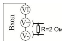
Рисунок 6 – Схема подключения датчика с токовым выходом (4-20) мА
